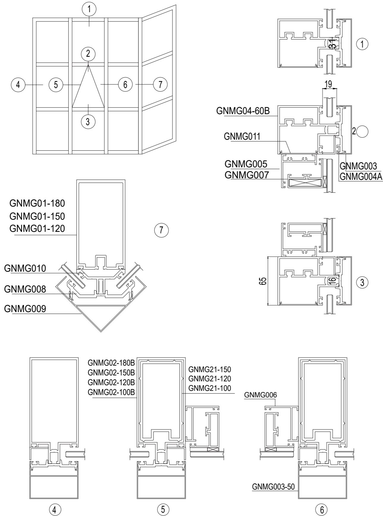
GNMG120、150、180、系列明框玻璃幕墙结构图
